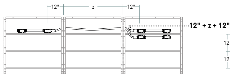
2 faisceaux doubles installés sur des traverses au même niveau
