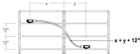
2 faisceaux simples installés au bout et au centre des cadres de base sur des traverses à différents niveaux
