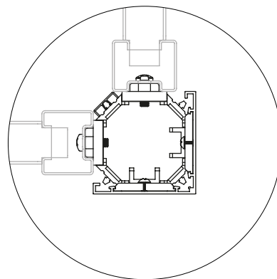
Connecteur « L » - 2 panneaux à 90°
