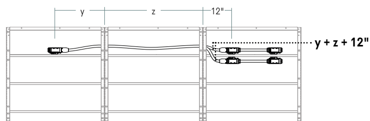
1 faisceau simple installé au centre d'un cadre de base et 1 faisceau double installé sur une traverse au même niveau
