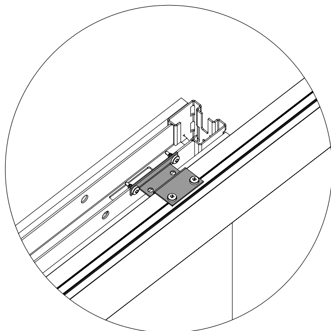
Installé sur un cadre superposable
