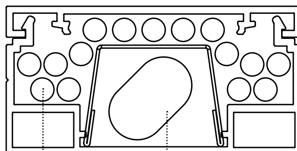
Colonnette 1 ½" x 3" - avec diviseur
