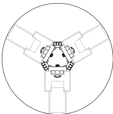
Connecteur « Y » - 3 panneaux à 120°
