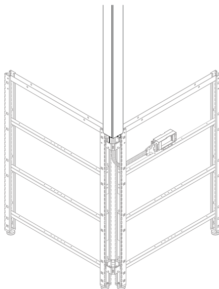
Colonnette d'alimentation de jonction
