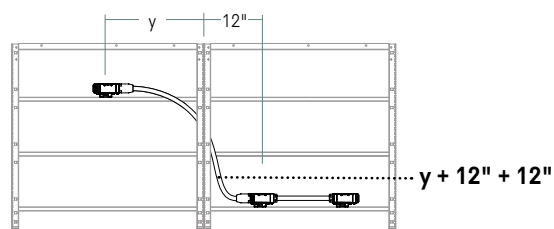
1 faisceau simple installé au centre d'un cadre de base et 1 faisceau double installé sur des traverses à différents niveaux
