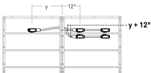
1 faisceau simple installé au centre d'un cadre de base et 1 faisceau double installé sur une traverse au même niveau
