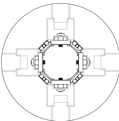
Connecteur « X » - 4 panneaux à 90°
