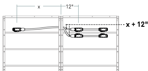
1 faisceau simple installé au bout d'un cadre de base et 1 faisceau double installé sur une traverse au même niveau
