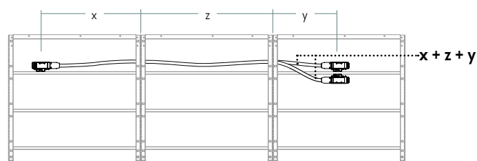
2 faisceaux simples installés au bout et au centre des cadres de base sur des traverses au même niveau
