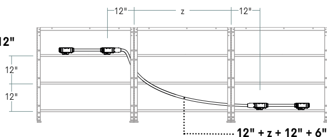
2 faisceaux doubles installés sur des traverses à différents niveaux
