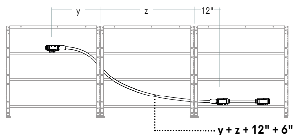
1 faisceau simple installé au centre d'un cadre de base et 1 faisceau double installé sur des traverses à différents niveaux.
