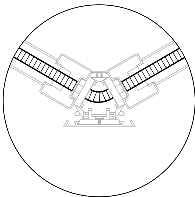
« V » 2 panneaux à 120°
