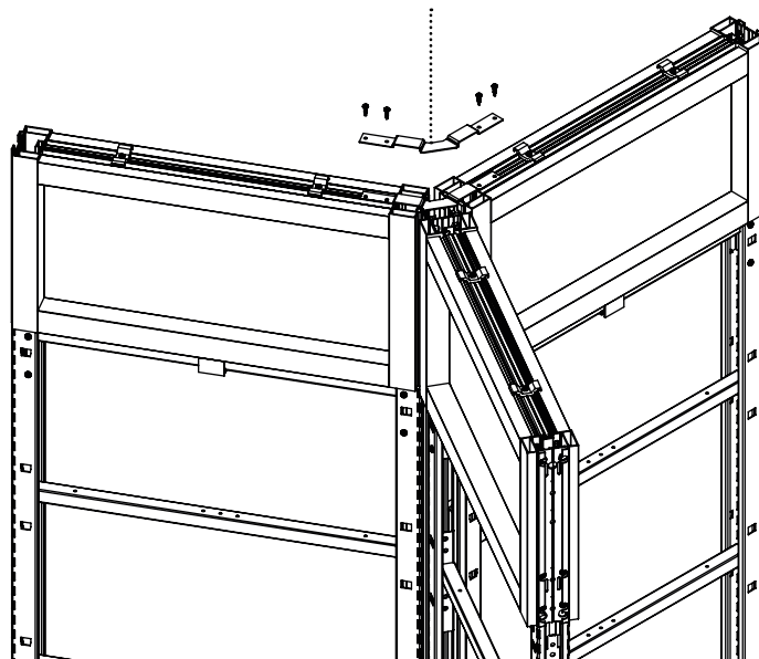
Attache de jonction « Y » FT-AJOGY
