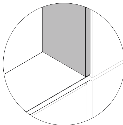
DÉTAIL B - GHxxC Enjoliveur de bout superposable « C » utilisé en fin de rangée lors de changement de hauteur (- long)
