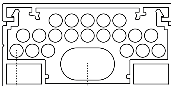
Colonnette 1 ½" x 3"
