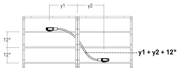
2 faisceaux simples installés au centre des cadres de base sur des traverses à différents niveaux
