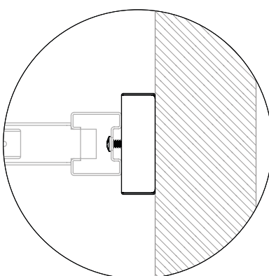
Connecteur « W » mural
