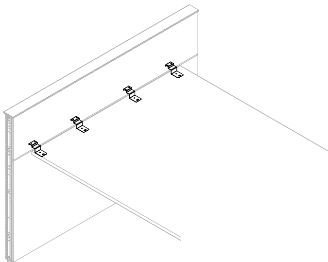
Surfaces de 48" Nombre de support hors module : 4
