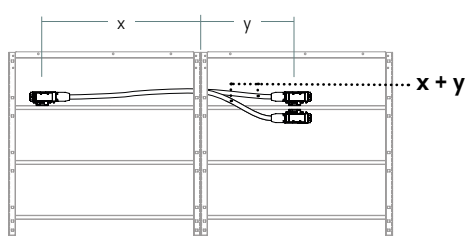
2 faisceaux simples installés au bout et au centre des cadres de base sur des traverses au même niveau
