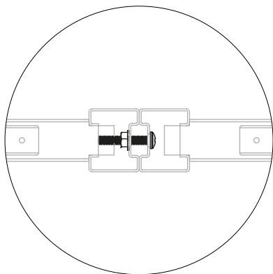
Connecteur « S » droit
