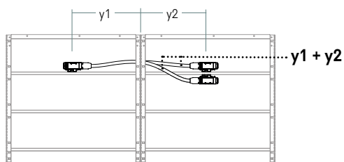
2 faisceaux simples installés au centre des cadres de base sur des traverses au même niveau
