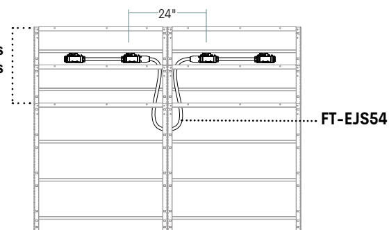
2 faisceaux doubles installés dans des cadres superposables au même niveau
