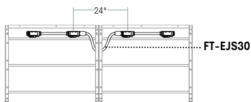
2 faisceaux doubles installés dans des cadres superposables au même niveau
