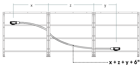
2 faisceaux simples installés au bout et au centre des cadres de base sur des traverses à différents niveaux
