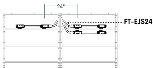
2 faisceaux doubles installés sur des traverses au même niveau
