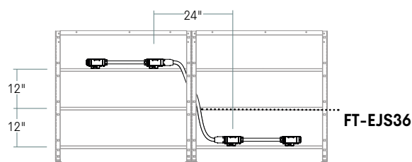
2 faisceaux doubles installés sur des traverses à différents niveaux
