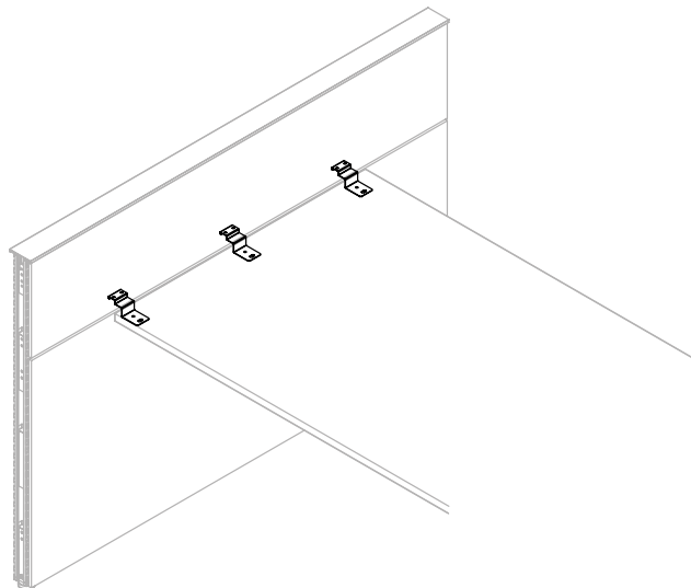
Surfaces de 36" et 42" Nombre de support hors module : 3
