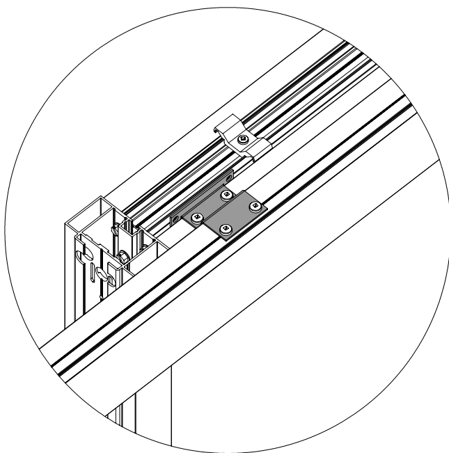
Installé sur un panneau superposable vitré
