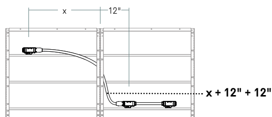
1 faisceau simple installé au bout d'un cadre de base et 1 faisceau double installé sur des traverses à différents niveaux
