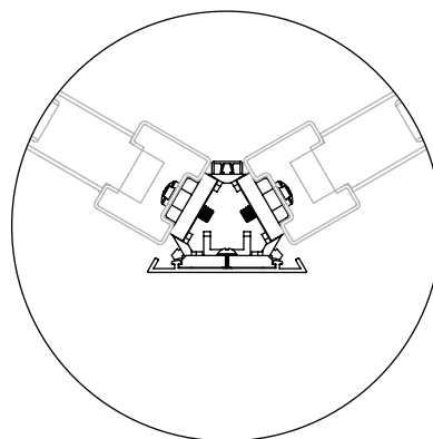
Connecteur « V » - 2 panneaux à 120°
