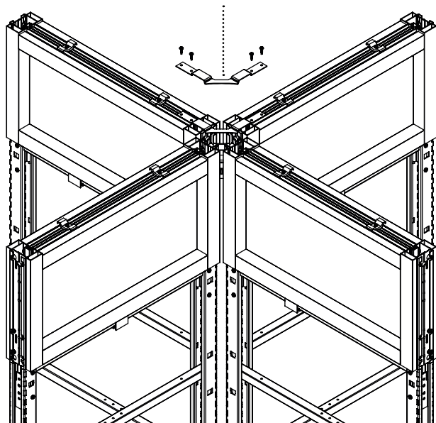
Attache de jonction « X » FT-AJOGX
