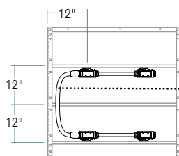
2 faisceaux installés sur des traverses à différents niveaux
