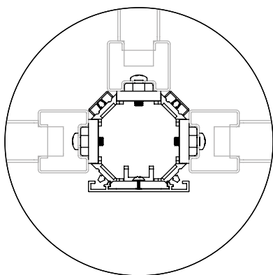
Connecteur « T » - 3 panneaux à 90°
