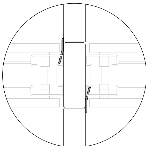
Panneaux latéraux accrochés - Gauche
