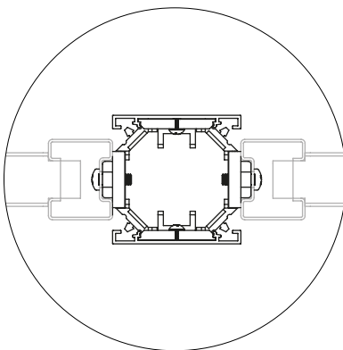
Connecteur « B » - 2 panneaux à 180°
